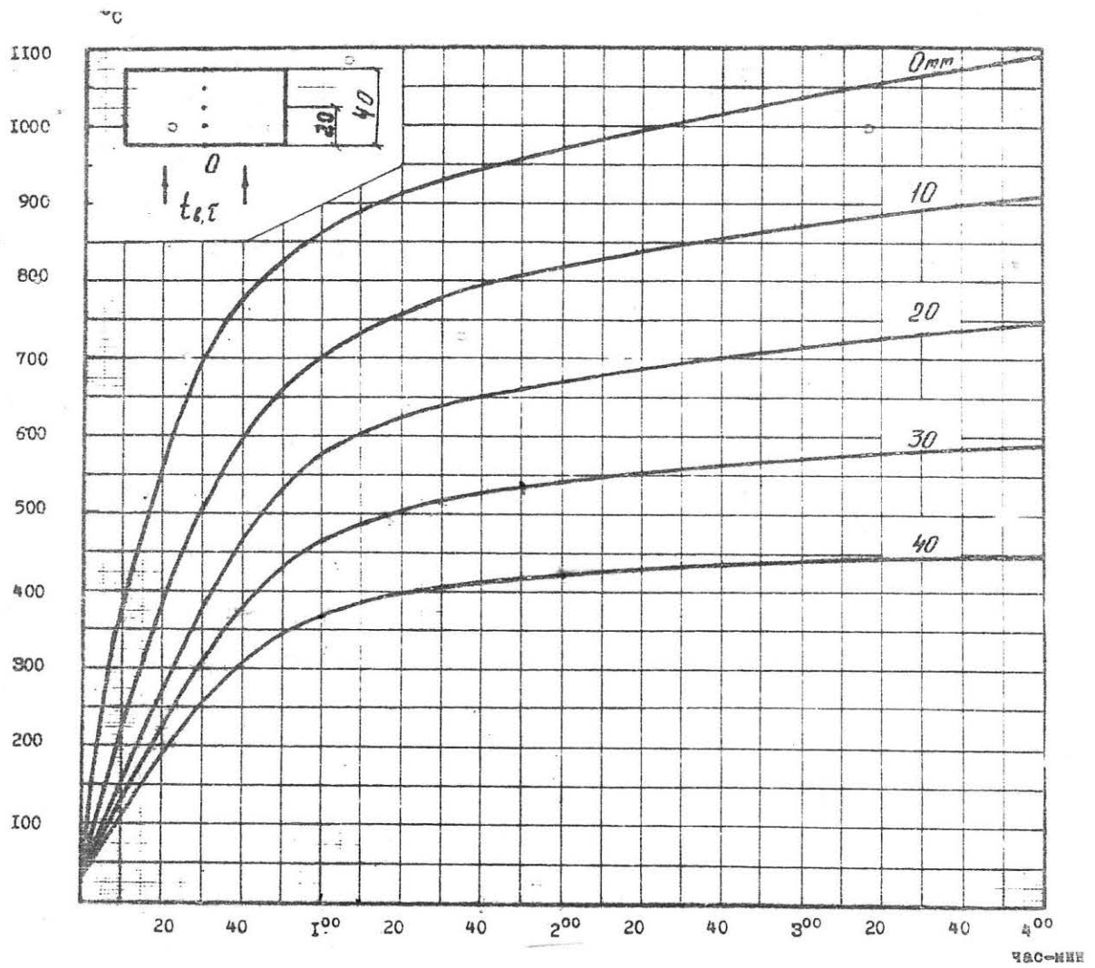
Рис. В.3. Прогрев необогреваемой поверхности сплошной плиты толщиной соответственно 40 мм из тяжелого бетона (плотность – 2330 кг/м 3 , влажность – 2,0 %) на гранитном заполнителе
