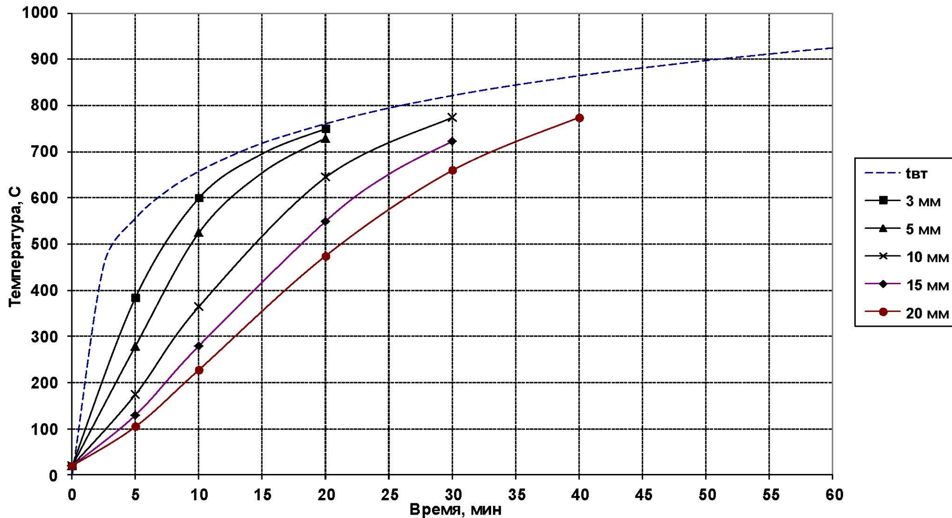
Рис. 1. Номограммы прогрева незащищенных стальных конструкций
