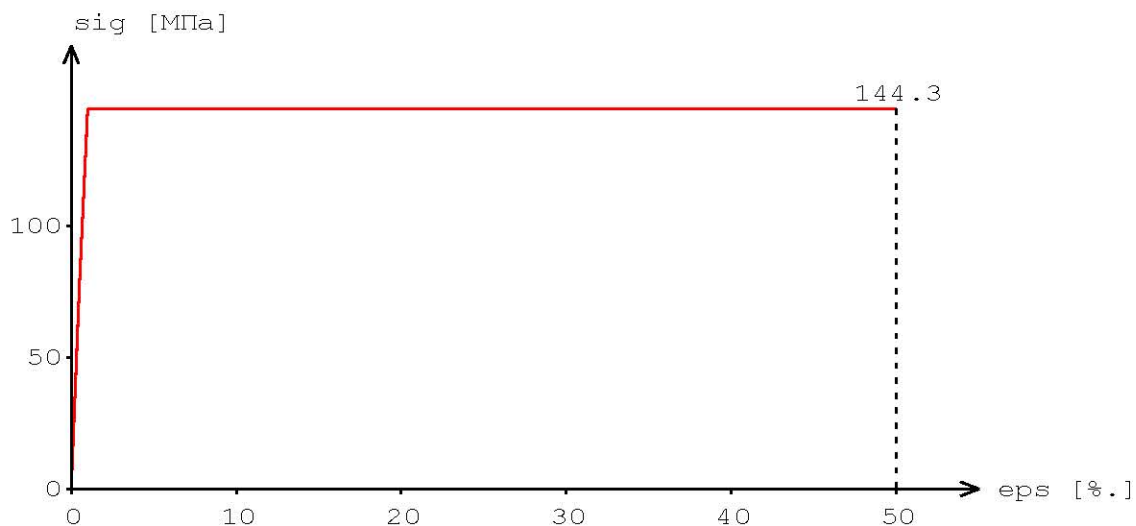
Рис. В.7. Диаграмма деформирования s-е стали при температуре 600 °С
