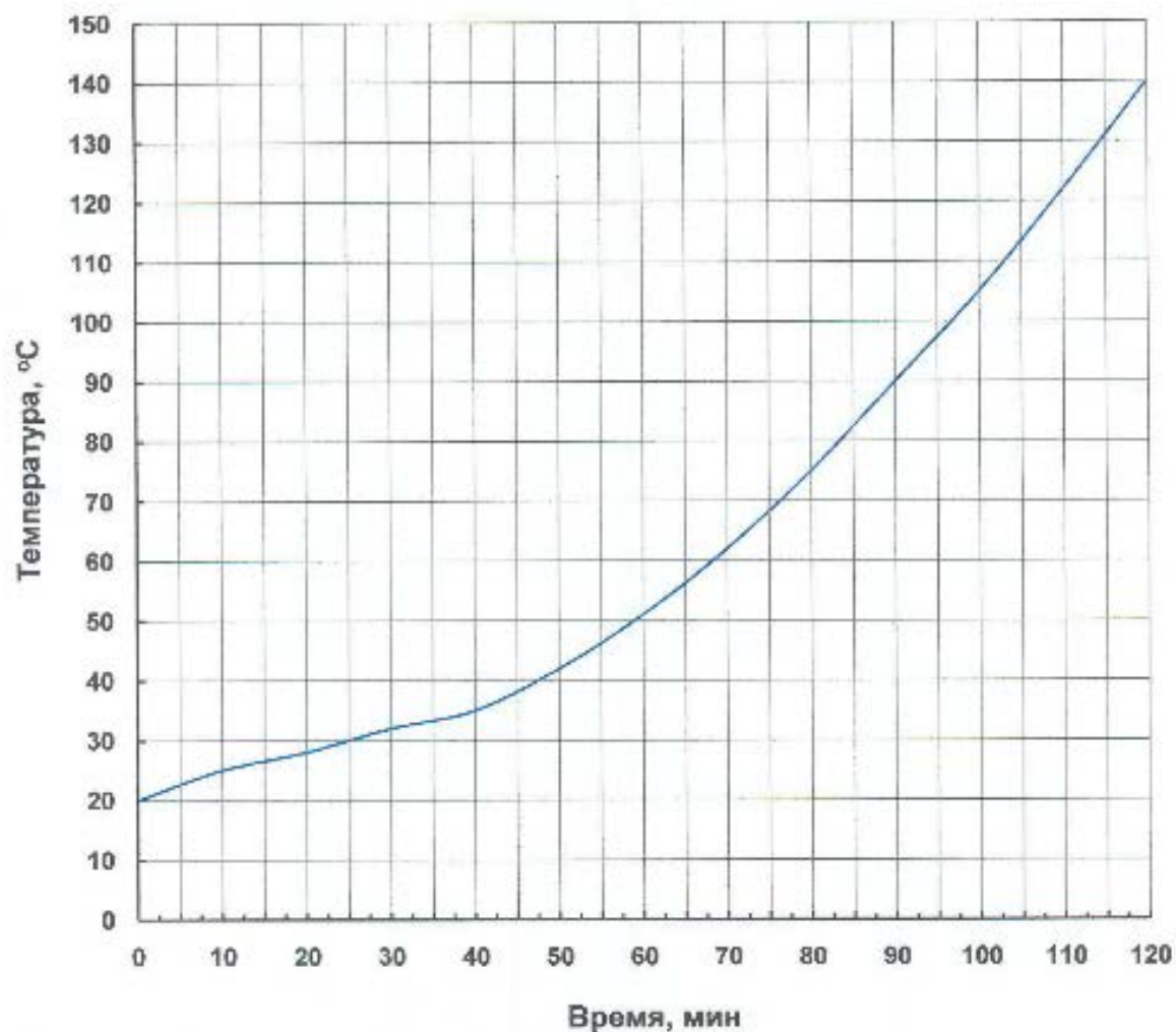
Рис. В.2. Прогрев необогреваемой поверхности сплошной и многопустотной плиты толщиной соответственно 120 и 160 мм из тяжелого бетона (плотность – 2330 кг/м 3 , влажность – 2,0 %) на гранитном заполнителе
