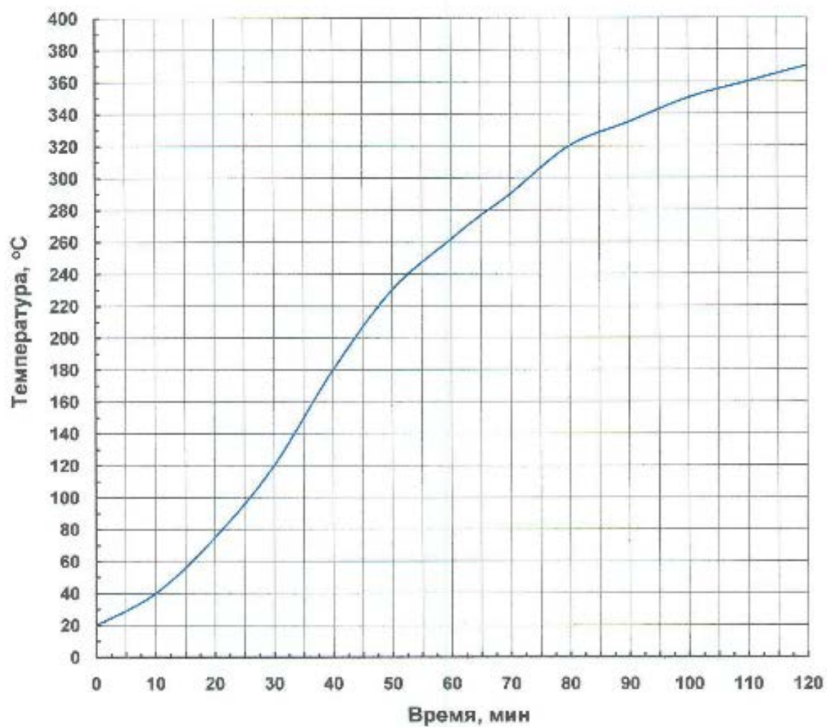
Рис. В. 1. Прогрев необогреваемой поверхности сплошной плиты толщиной 50 мм из тяжелого бетона (плотность – 2330 кг/м 3 , влажность – 2,0%) на гранитном заполнителе
